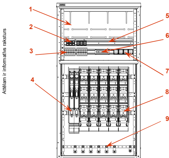
2. att. Aparatūras un elementu izvietojums
