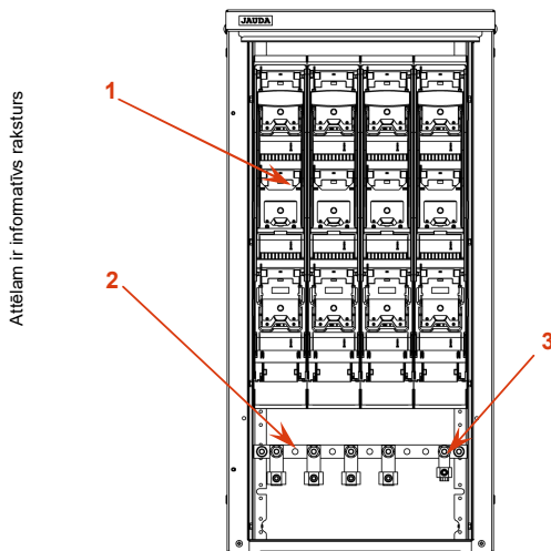
2. att. Aparātūras un elementu izvietojums
