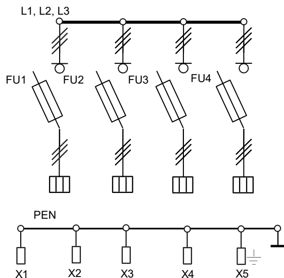
1. att. Elektriskā principshēma
